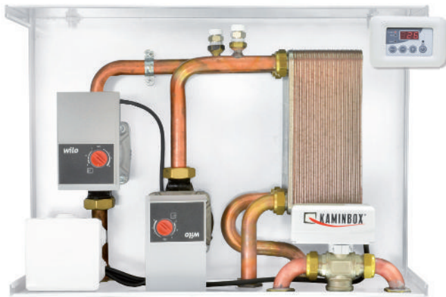
DIMENSIONI: 16 x 49,5 x 34 cm (PxBxH)
